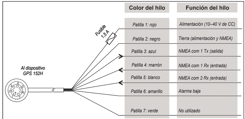
Arnés de cableado del dispositivo GPS 152H
